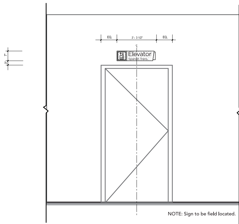
8 ELEVATION SCALE: 1/2" = 1' - 0"
