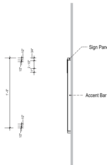
3 SIDE VIEW SCALE: 1 - 1/2" = 1' - 0"
