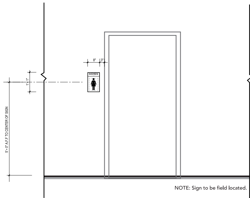
7 ELEVATION SCALE: 1/2" = 1' - 0"
