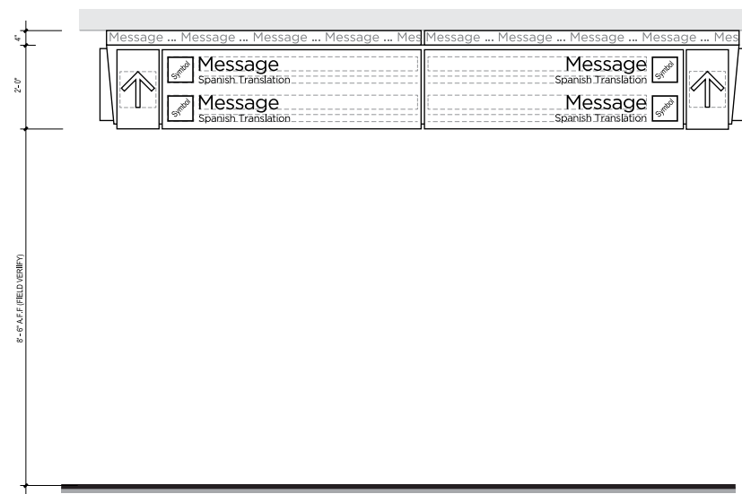
6 ELEVATION SCALE: 1/2" = 1' - 0"
