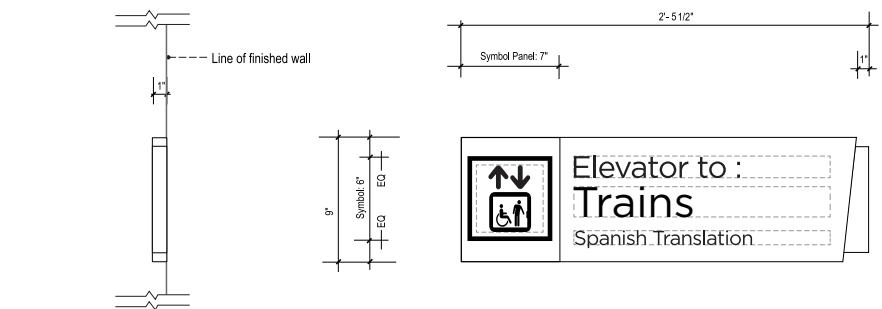
3 SIDE VIEW SCALE: 1-1/2" = 1' - 0"
