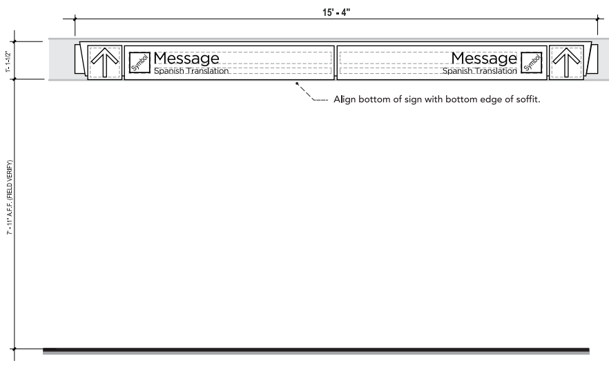
6 ELEVATION SCALE: 1/2" = 1' - 0"
