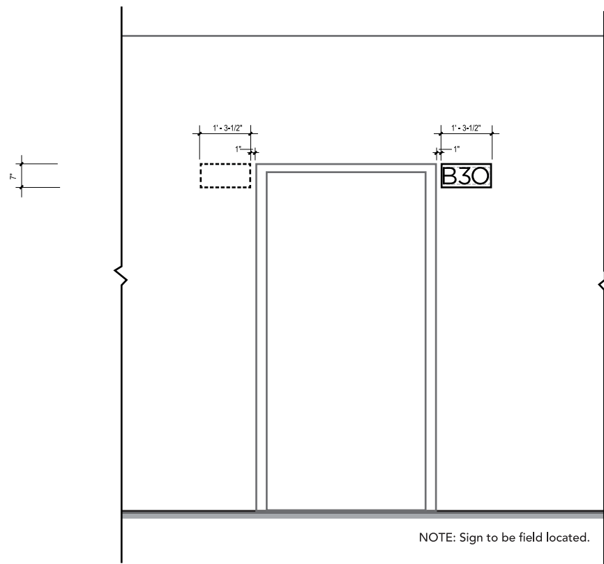
5 ELEVATION SCALE: 1/2" = 1' - 0"
