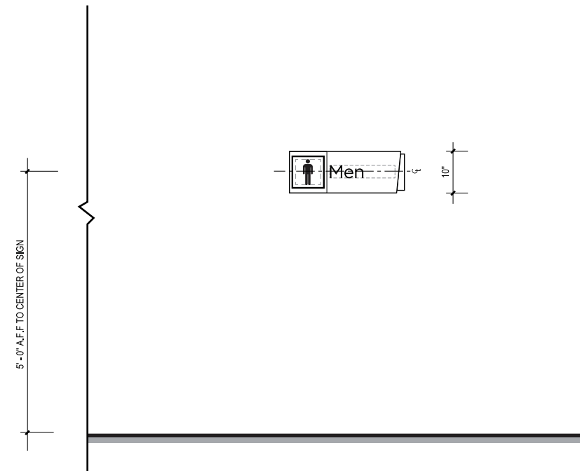
9 ELEVATION SCALE: 1 - 1/2" = 1' - 0"
