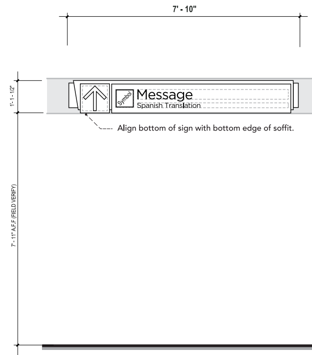
6 ELEVATION SCALE: 1/2" = 1' - 0"
