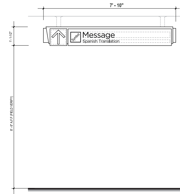
6 ELEVATION SCALE: 1/2" = 1' - 0"
