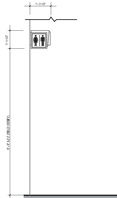
8 ELEVATION SCALE: 1-1/2" = 1' - 0"
